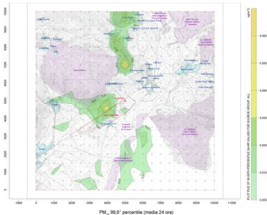
Figura 8.3.7d 99,6° percentile PM_{10}
