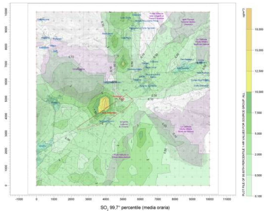
Figura 8.3.7e 99,7° percentile SO 2
